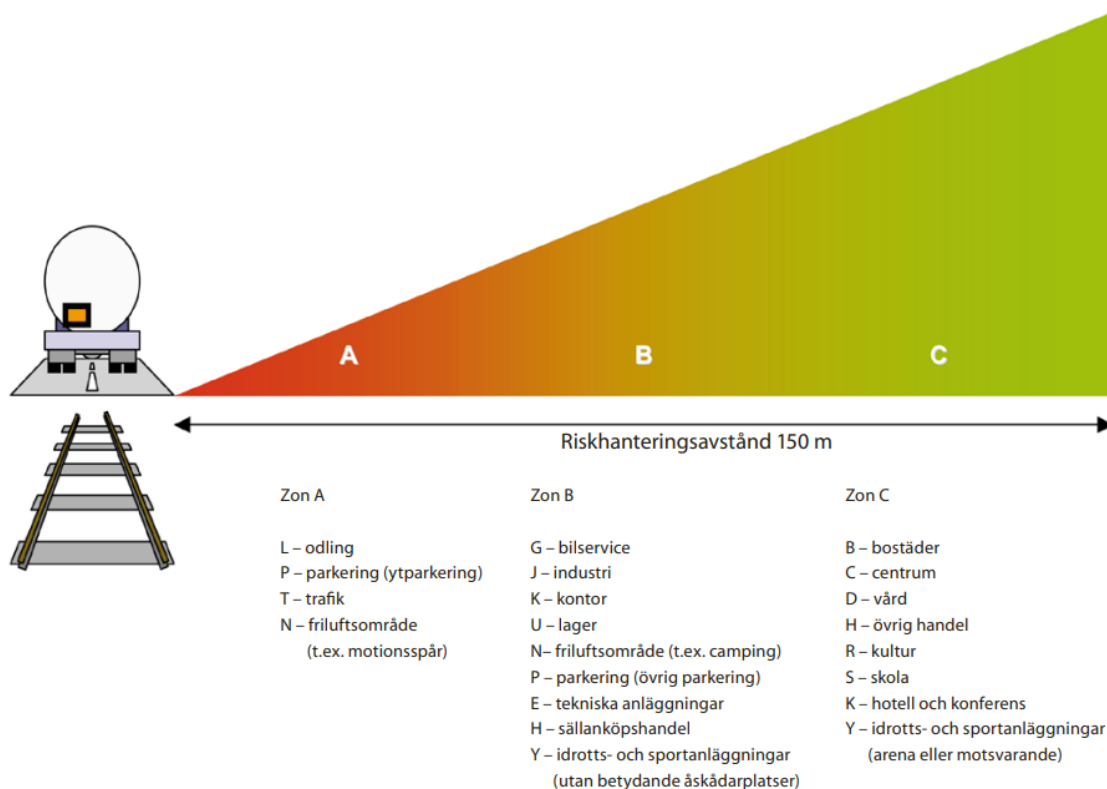
Figur 15. Zonindelning för länsstyrelsernas riskpolicys riskhanteringsavstånd. Från Riskhantering i detaljplaneprocessen – riskpolicy för markanvändning intill transportleder för farligt gods , 2006.
