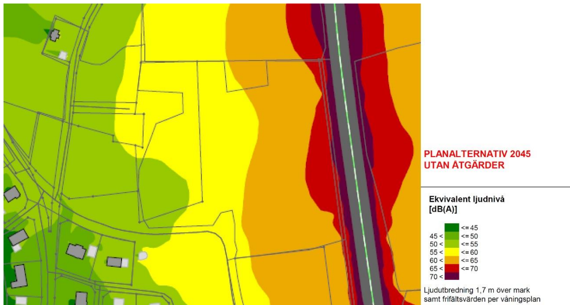
Figur 7. Den gröna och gula ytan tyder på att planlagd kvartersmark 2045 beräknas ha en ekvivalent ljudnivå på max 55 respektive 60 dBA. Utdrag från bilaga för Norconsult AB:s utredning PM Trafikbullerutredning – E20 Vårgårda – Norr Mariestad etapp Förbi Skara, delen Vilan-Dalaån – E20 Vårgårda – Norr Mariestad, etapp Förbi Skara, delen Dalaån-Ledsjö , 2016-08-25.
