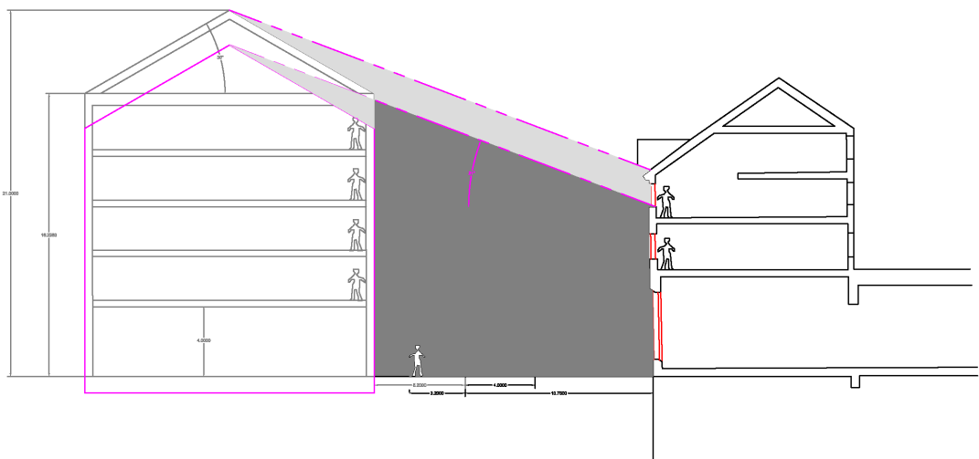
Figur 19- Vintertid sker ingen skuggning. Under höst och vårdagjämning 23 sept (kl.9-15) samt 20 mars (kl.10-16) när solvinkeln är över 21 grader sker en viss extra beskuggning av planändringen som påverkar ett dagsljuset under 1 h på förmiddagen och en timme på eftermiddagen.
