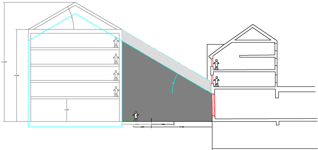
Figur 18 - Midsommar kl.8-18 och april/augusti (kl.10-15) när solvinkeln är minst 35 grader. sker ingen extra beskuggning av planändringen. Lägre solvinklar kan dock påverka något på morgon och sen eftermiddag..
