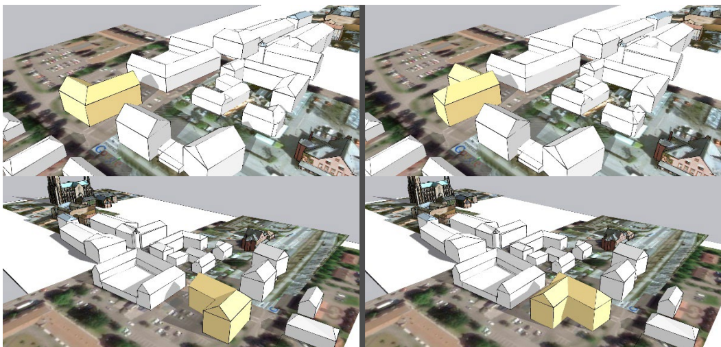
Bild över placering av byggnad till vänster som uppfyller planbestämmelsen samt överstrukna bilder till höger med placering av byggnad som inte uppfyller bestämmelsen då en av långsidorna är mot GC-väg och inte Gågatan (Klostergatan) eller Huvudgata (Vallgatan).
