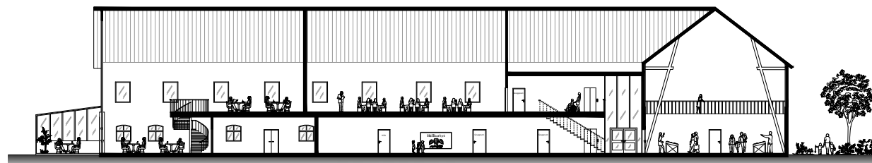
Sektion A-A Skala 1:200 (A3)
